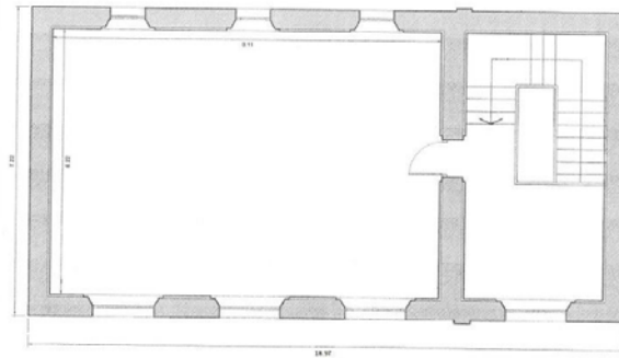
Planta Primera
