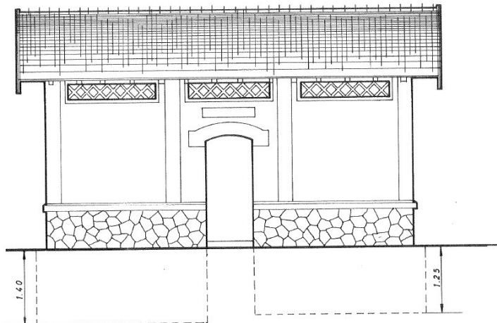
FACHADA LATERAL
