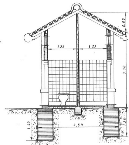
SECCION A-B
