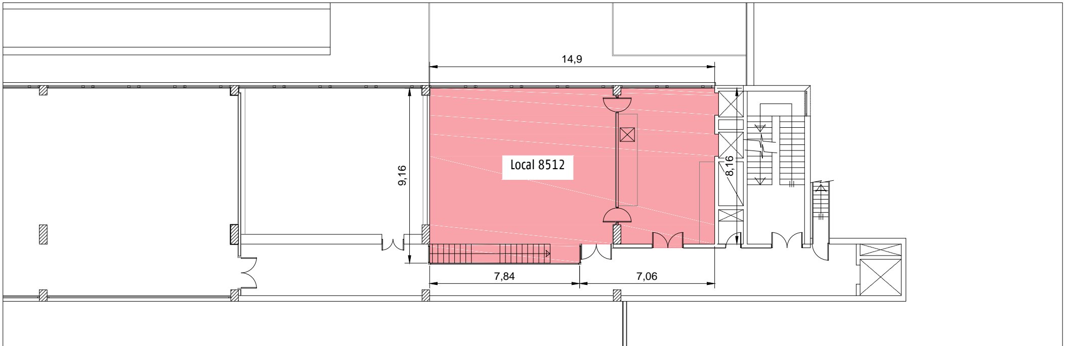
DETALLE LOCAL 8512. PLANTA ALTA
