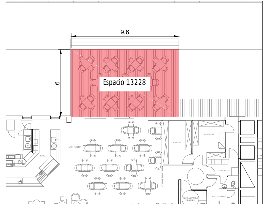
DETALLE ESPACIO 13228. PLANTA BAJA
