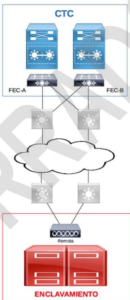
Esquema de arquitectura simple.
