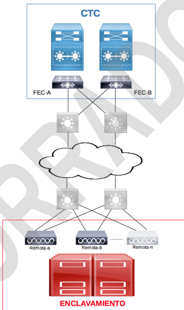
Esquema de arquitectura redundante
