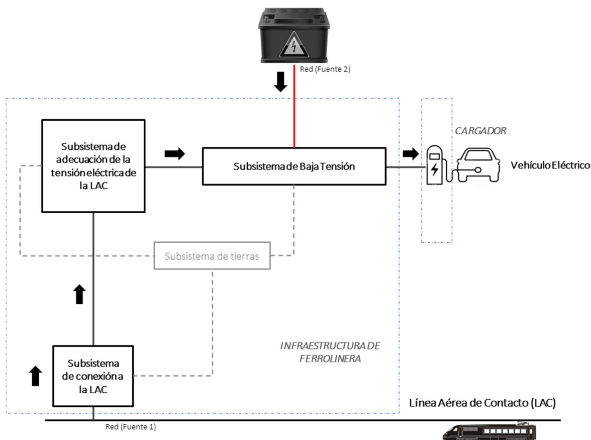
Figura 2. Alimentación redundante
