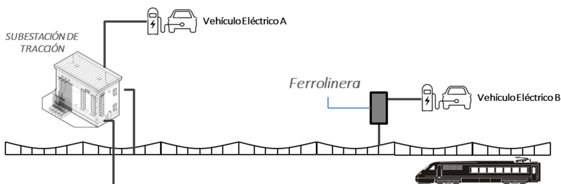
Figura 1. Conexión posible de la estación de recarga de vehículos eléctricos a la red eléctrica ferroviaria: Conexión directa a la subestación de tracción o conexión directa a la Línea Aérea de Contacto.
