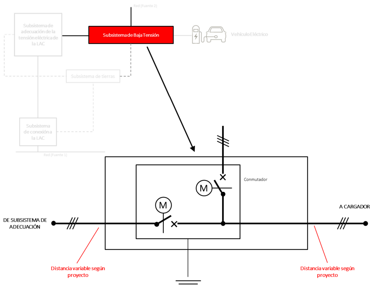
Figura 4. . Esquema general (abreviado) asociado al subsistema de Baja Tensión (de 3 kV CC).
