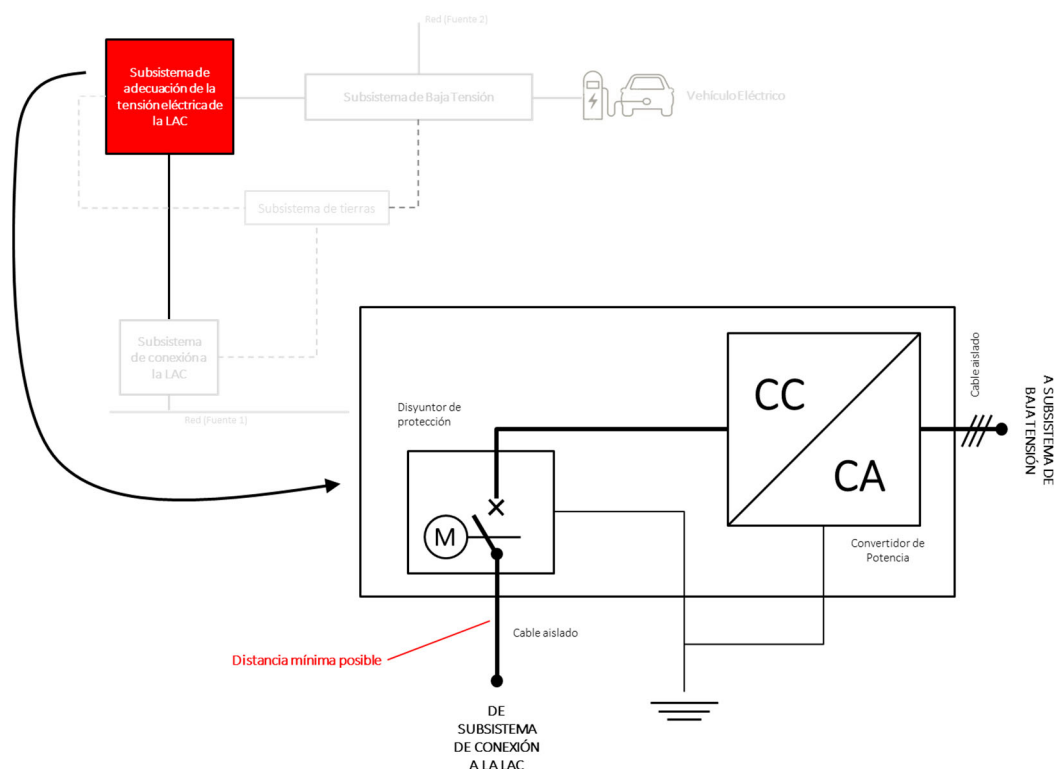
Figura 4. . Esquema general (abreviado) asociado al subsistema de adecuación a la LAC (de 3 kV CC).
