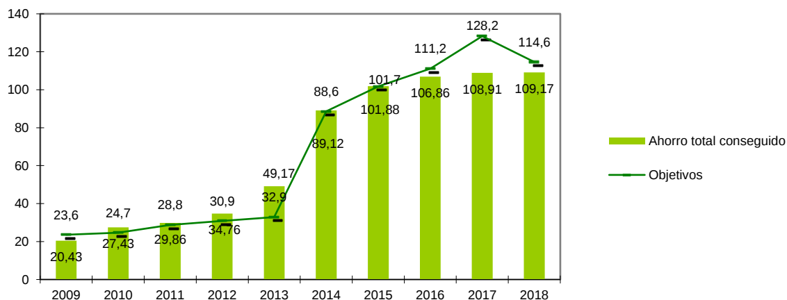
Gráfico 9. Realizaciones a 31 de diciembre de cada año de los Planes de Implantación de Acciones de Ahorro y Eficiencia Energética y Sistemas de Generación de Energía Renovable, en Adif y Adif-Alta Velocidad. Ahorro total conseguido y objetivos (GWh/año)
