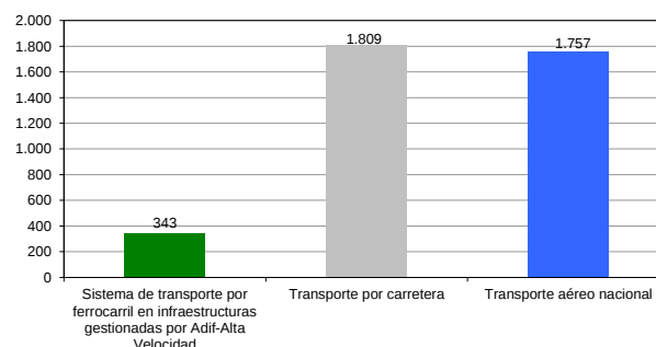
Gráfico 57. Consumo energético por UT (kJ/UT). Año 2017 (último año disponible). *
