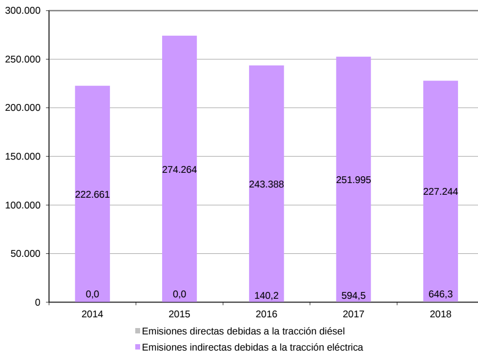
Gráfico 58. Emisiones de GEI derivadas de la tracción. Sistema de transporte por ferrocarril en infraestructuras gestionadas por Adif-Alta Velocidad (t de CO 2 eq/año)
