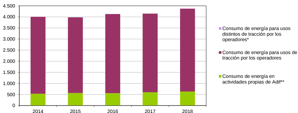
Gráfico 52. Consumo total de energía en el sistema ferroviario gestionado por Adif-Alta Velocidad (TJ/año)
