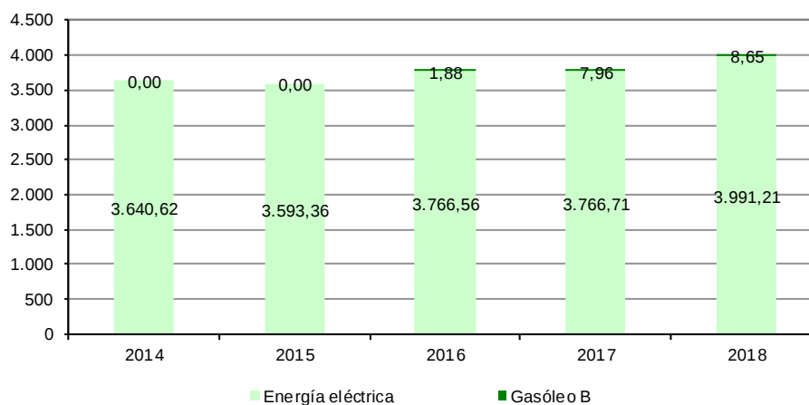
Gráfico 51. Consumo energético para usos de tracción (TJ/año) *
