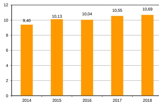
Gráfico 13. Intensidad energética final (MJ/km-tren gestionado)*
