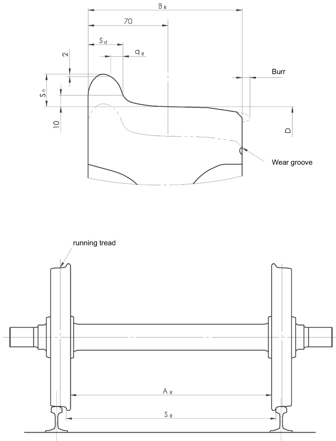
Figura 2: Dimensiones de la rueda y del juego de ruedas
